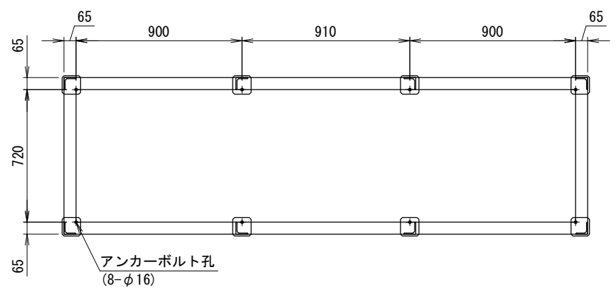
<アンカー寸法図> SCALE= 1:20
