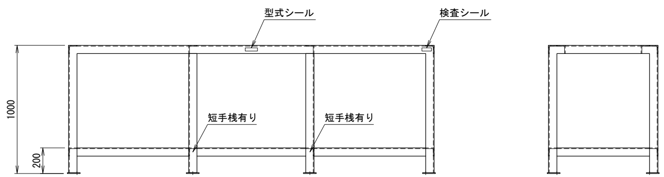
<アンカー寸法図> SCALE= 1:20
