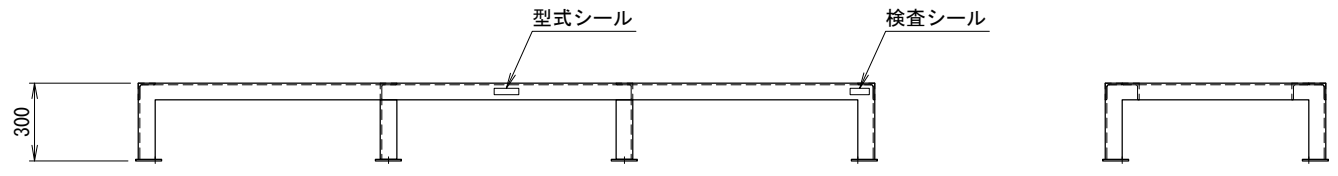
<アンカー寸法図> SCALE= 1:20
