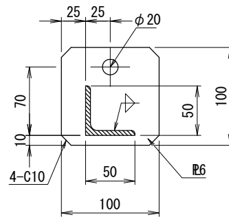
ロ部詳細
