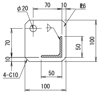
I部詳細
