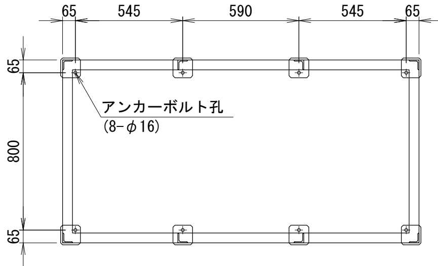
<アンカー寸法図> SCALE= 1:20
