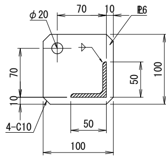
アンカー位置部詳細
