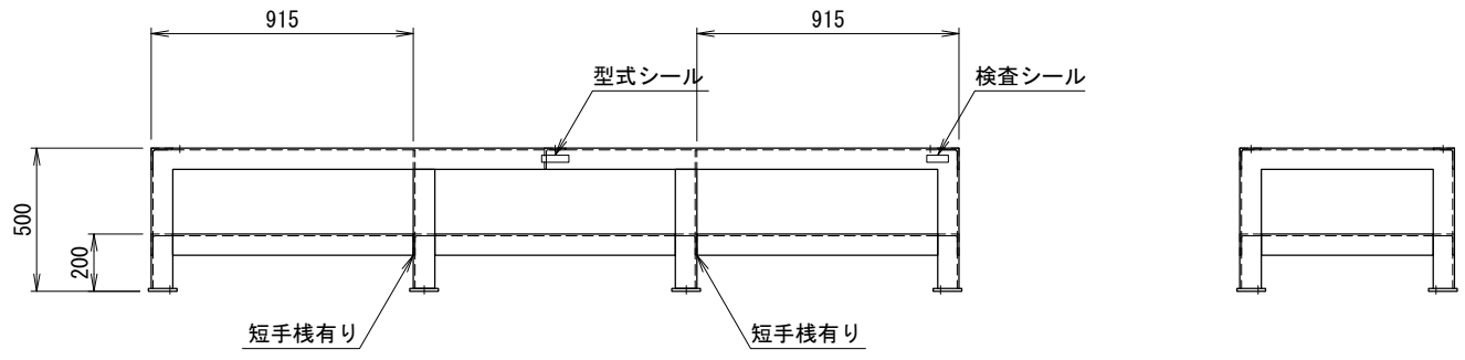
<アンカー寸法図> SCALE= 1:25
