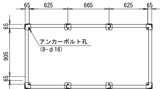
<アンカー寸法図> SCALE= 1:25
