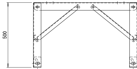
アンカー金具取付 (B)
