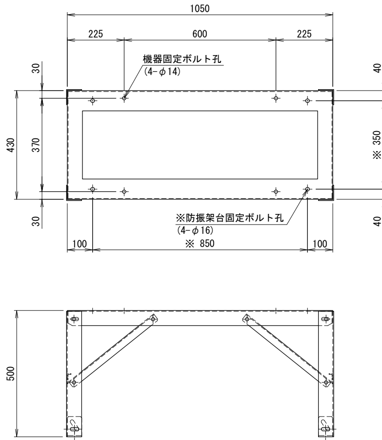
アンカー金具取付 (B)
