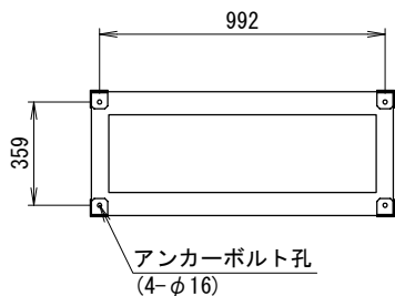
〈アンカー寸法図〉 SCALE= 1:20 アンカー金具取付 (A)
