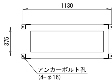
アンカー金具取付 (B)
