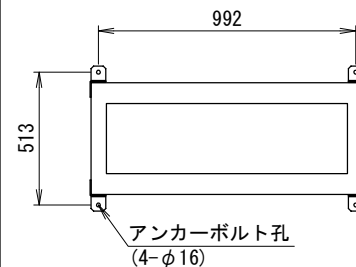
アンカー金具取付 (C)
