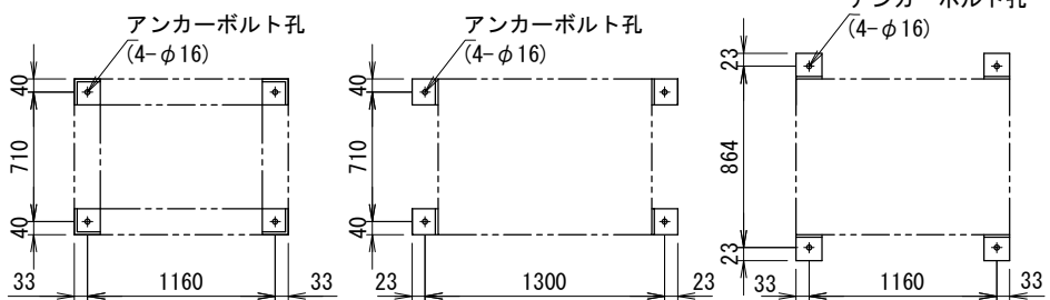
アンカー金具取付 (A)
