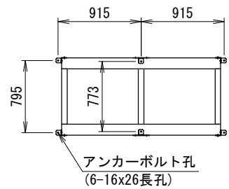
アンカー金具取付 (B) 外側側面
