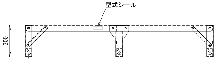
<アンカー寸法図(長孔中心)> SCALE= 1:40 アンカー金具取付 (A) 内側
