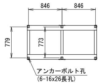
<アンカー寸法図(長孔中心)> SCALE= 1:40 アンカー金具取付 (A) 内側
