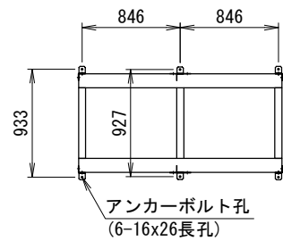
アンカー金具取付 (C) 外側前後面
