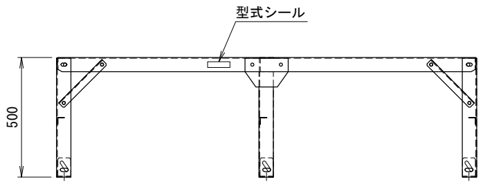
<アンカー寸法図(長孔中心)> SCALE= 1:40 アンカー金具取付(A)内側
