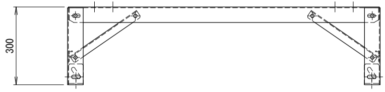
<アンカー寸法図> SCALE= 1:25 アンカー金具取付 (A)
