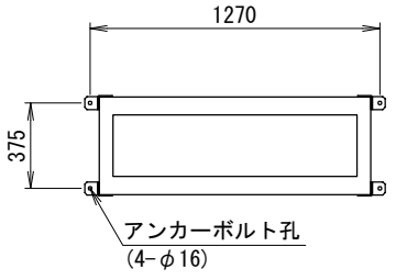
アンカー金具取付 (B)
