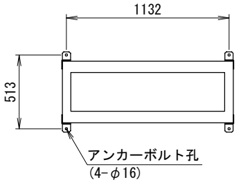
アンカー金具取付 (C)
