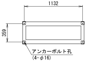
<アンカー寸法図> SCALE= 1:25 アンカー金具取付 (A)
