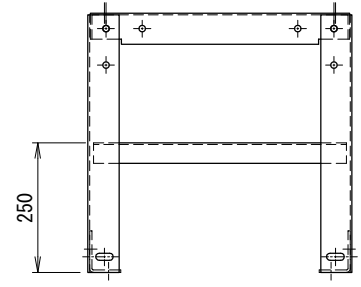
アンカー金具取付 (C)
