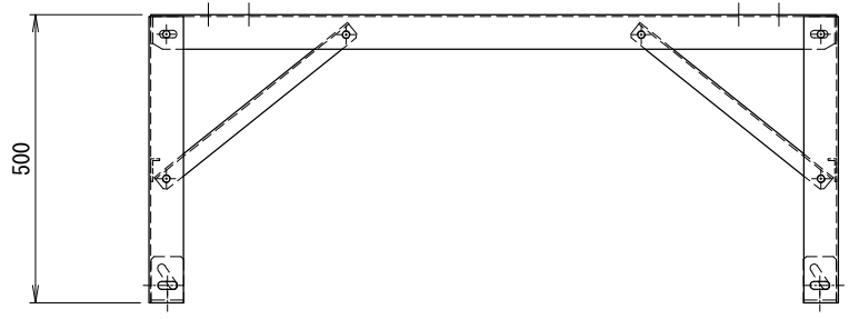
<アンカー寸法図> SCALE= 1:25 アンカー金具取付 (A)
