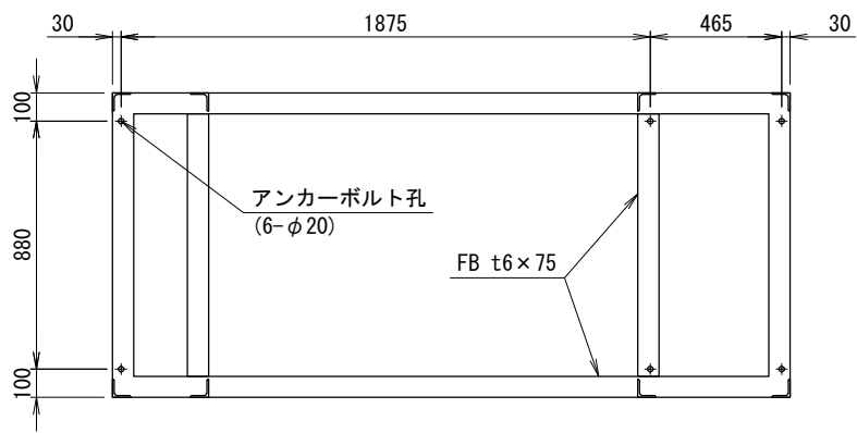
<アンカー寸法図> SCALE= 1:20
