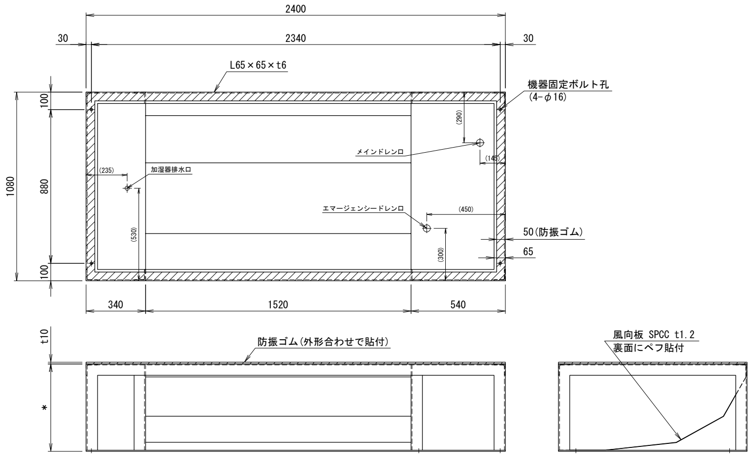
<アンカー寸法図> SCALE= 1:20
