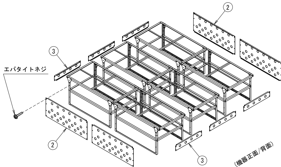
▲ パンチングプレート取付詳細図
