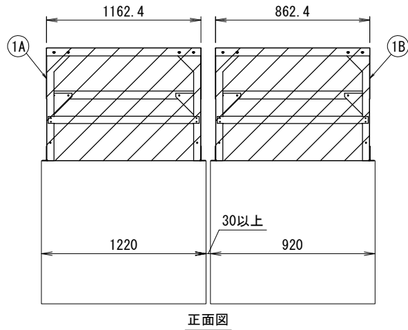
<防雪ルーフ配置寸法図>
