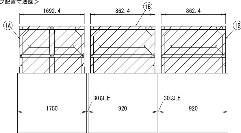
正面図
