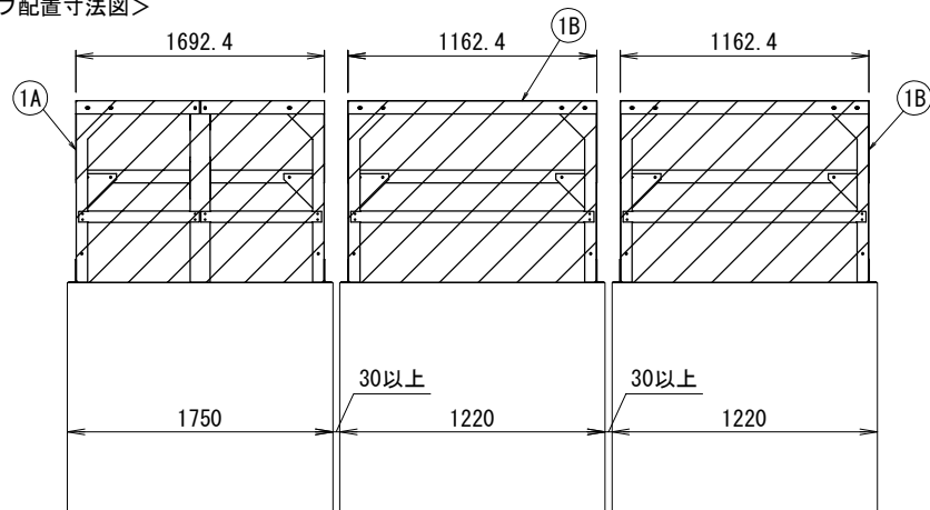
正面図
