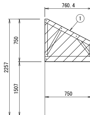
右側面図
