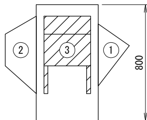
左側面図
