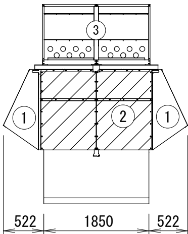
右側面図
