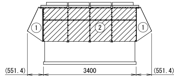
右側面図
