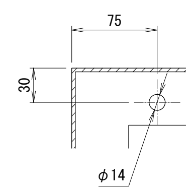
<アンカー部詳細> アンカーボルト参考 接着系アンカー : M10 有効埋め込み深さ : 80mm以上
