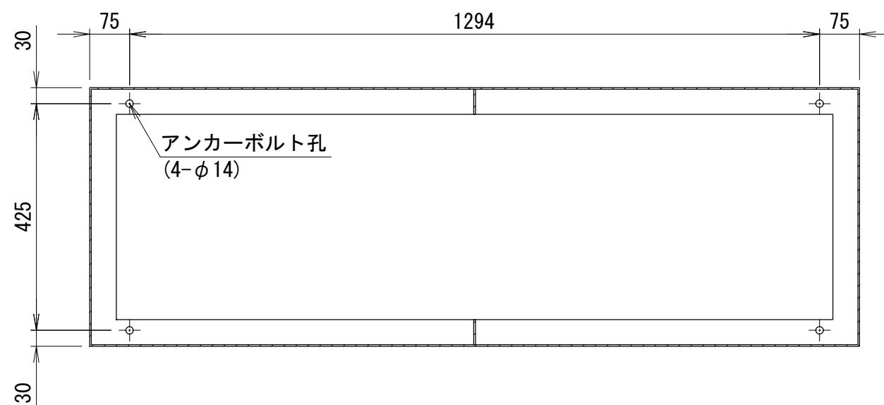
<アンカー寸法図> SCALE= 1:10
