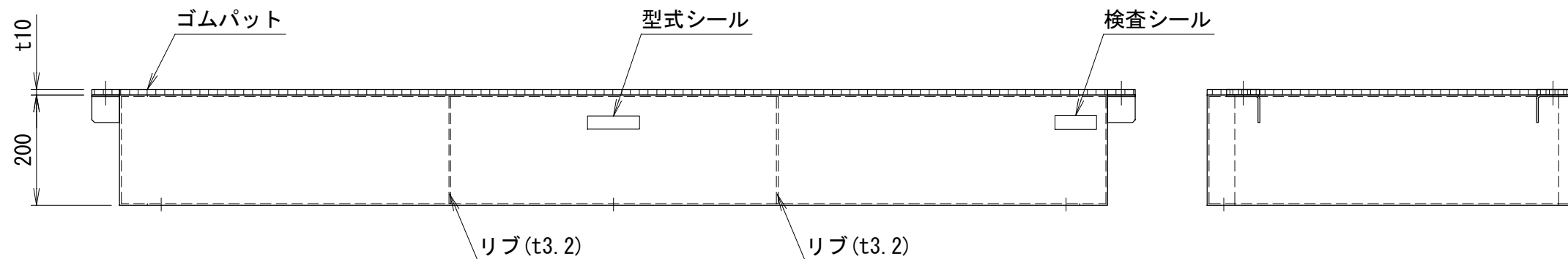
<アンカー寸法図> SCALE= 1:15
