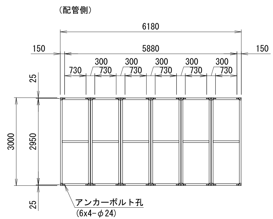
<アンカー寸法図 (下ベース基準) ※A孔>
