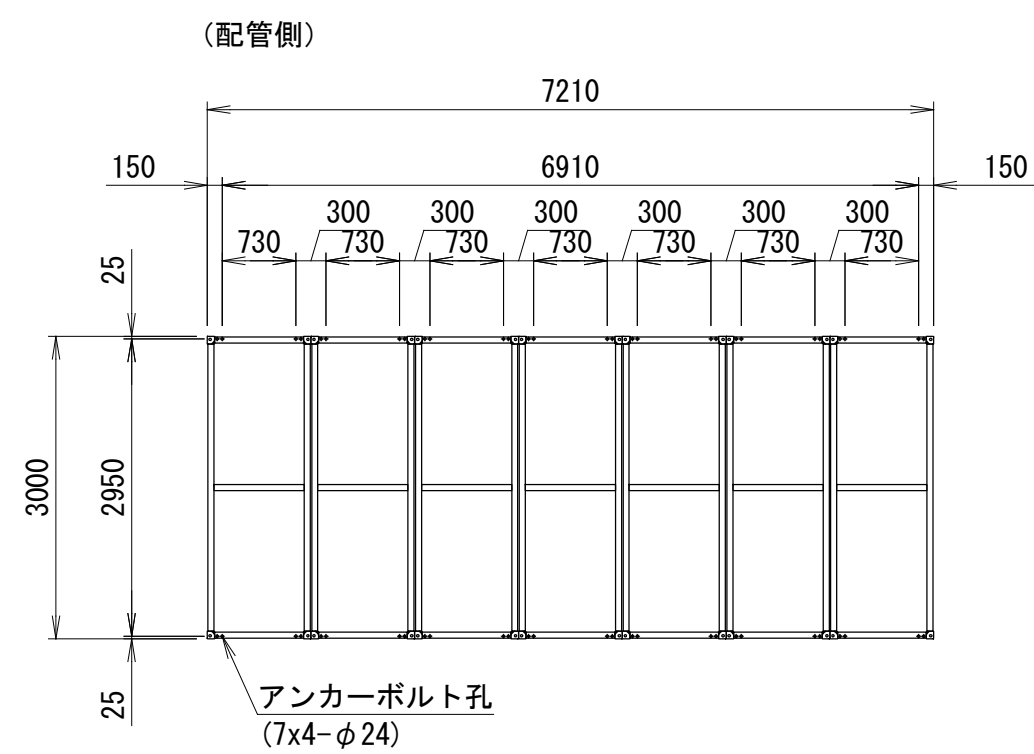
<アンカー寸法図 (下ベース基準) ※A孔>
