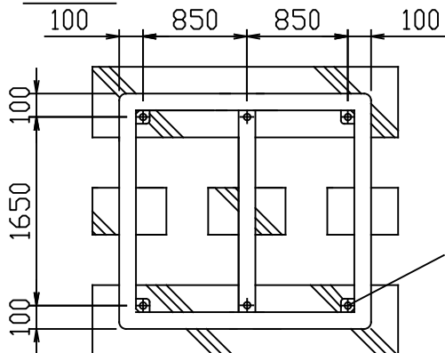
基礎図
