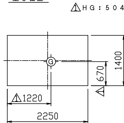
重心位置
