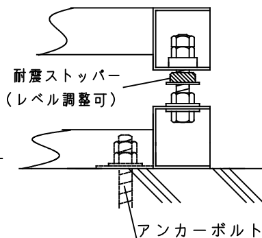
アンカー及びストッパー
