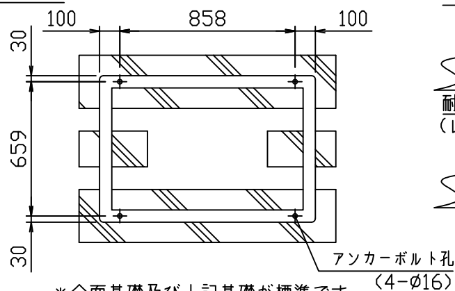
基礎図
