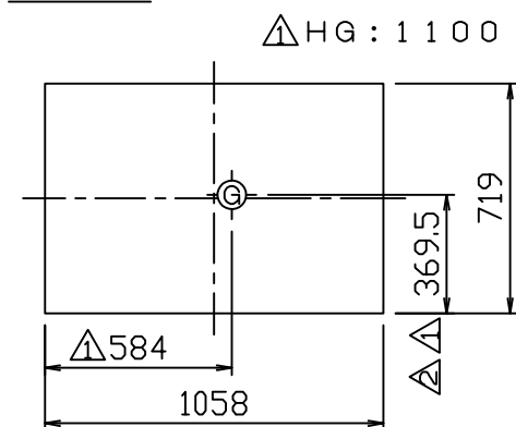
重心位置
