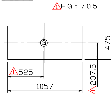
重心位置
