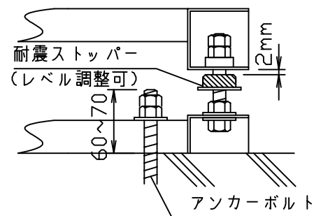
アンカー及びストッパー
