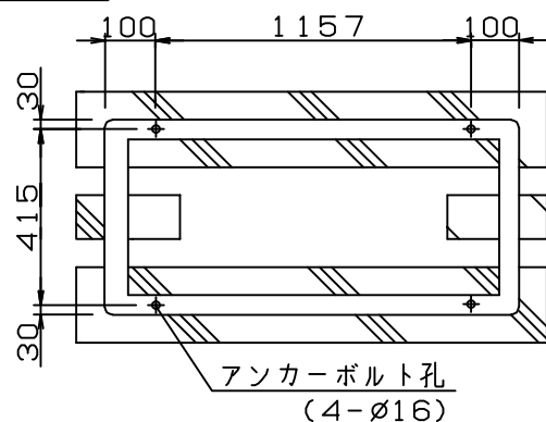
基礎図
