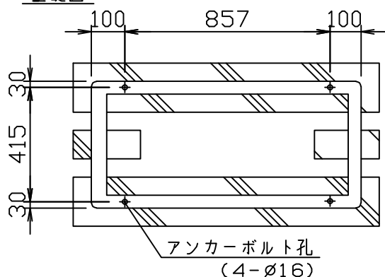
基礎図
