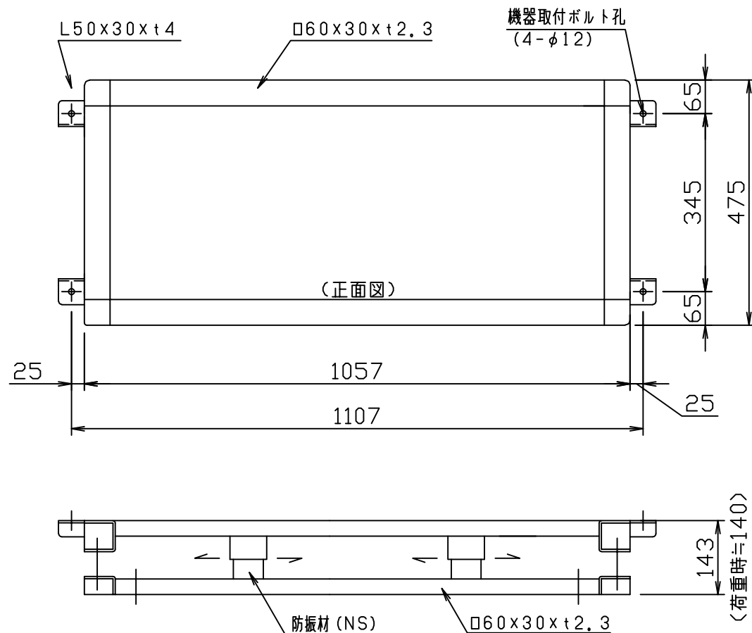
基礎図
