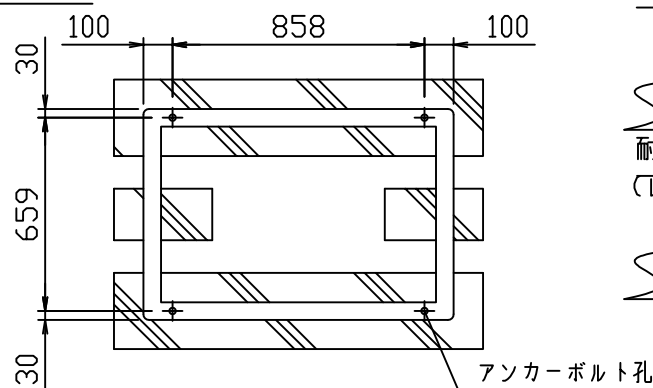
基礎図
