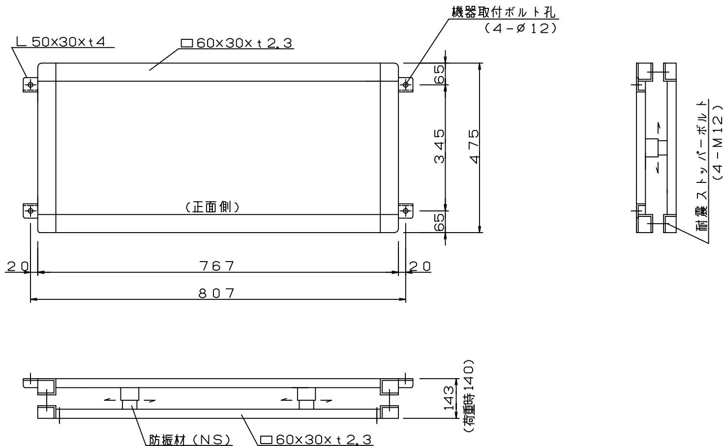
基礎図
