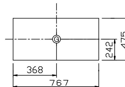
重心位置
