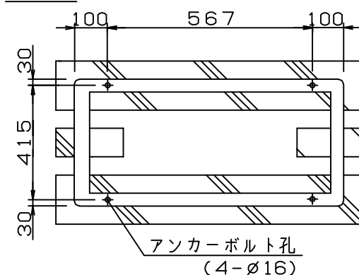
基礎図
