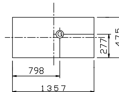
重心位置
