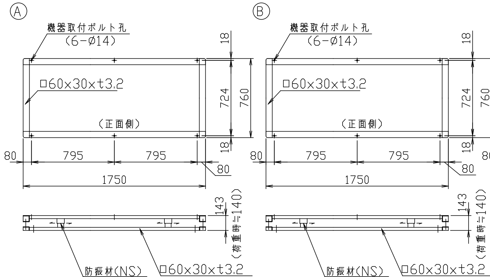
基礎図
