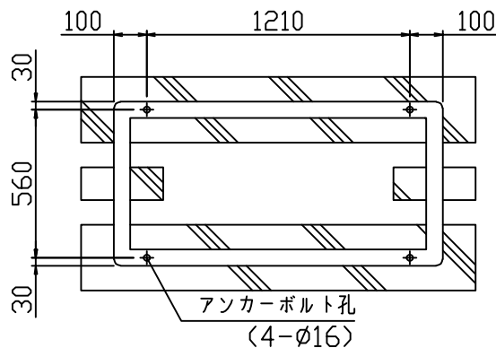
基礎図
