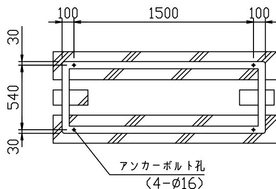
基礎図
