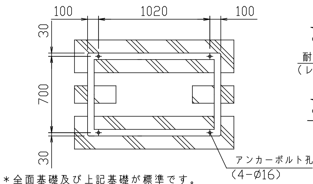
基礎図
