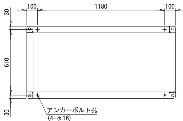
〈アンカー寸法図〉 SCALE= 1:15
