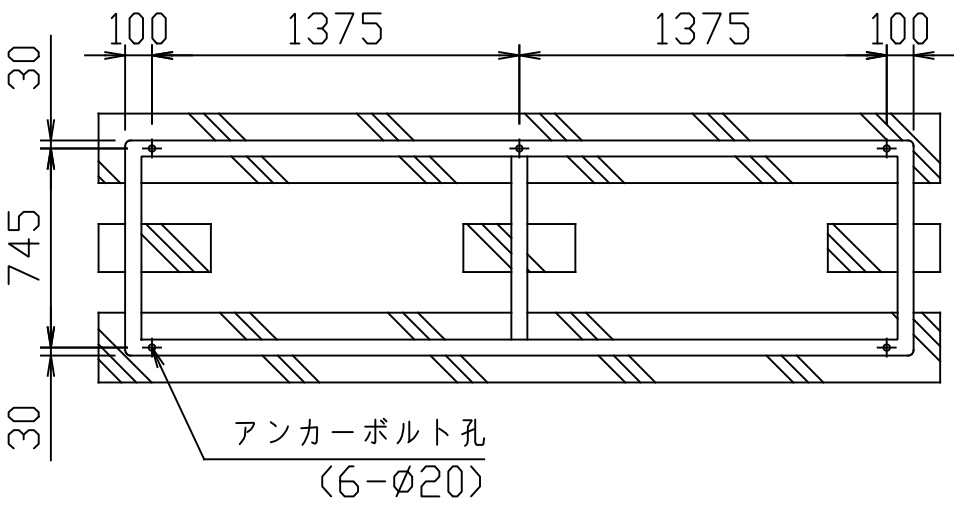
基礎図
