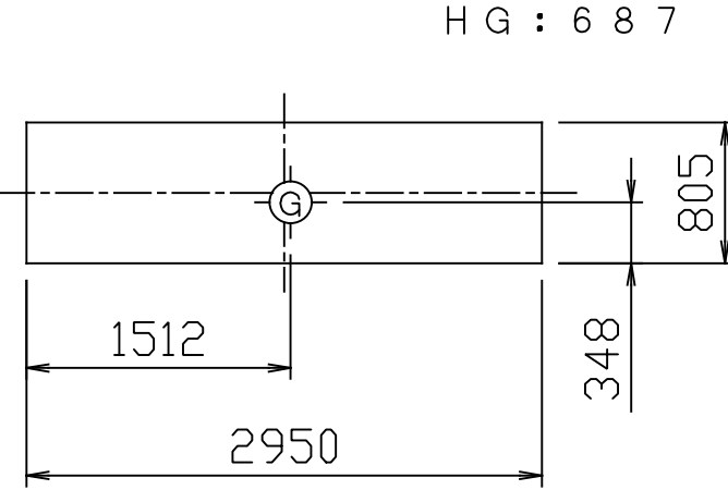
重心位置
