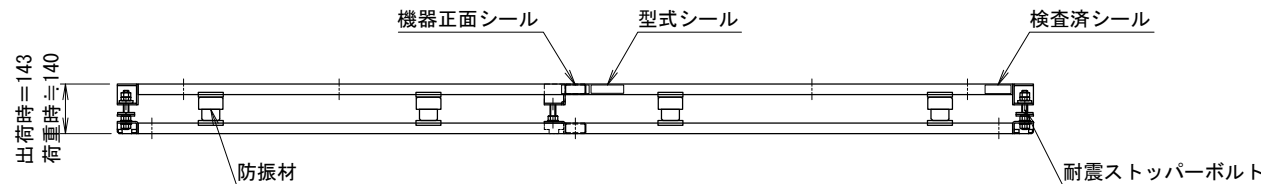
〈アンカー寸法図〉 SCALE= 1:20
