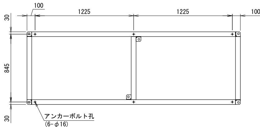
〈アンカー寸法図〉 SCALE= 1:20
