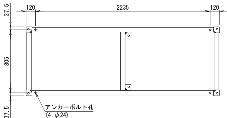
〈アンカー寸法図〉 SCALE= 1:20
