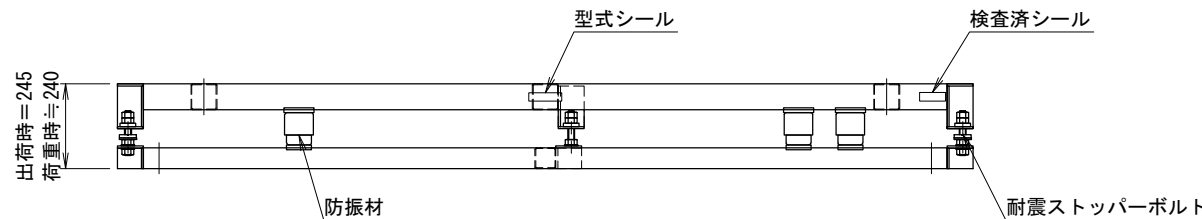
〈アンカー寸法図〉 SCALE= 1:20
