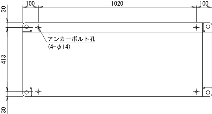
＜アンカー寸法図＞ SCALE= 1:10
