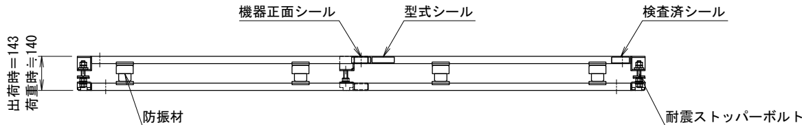
<アンカー寸法図> SCALE= 1:20
