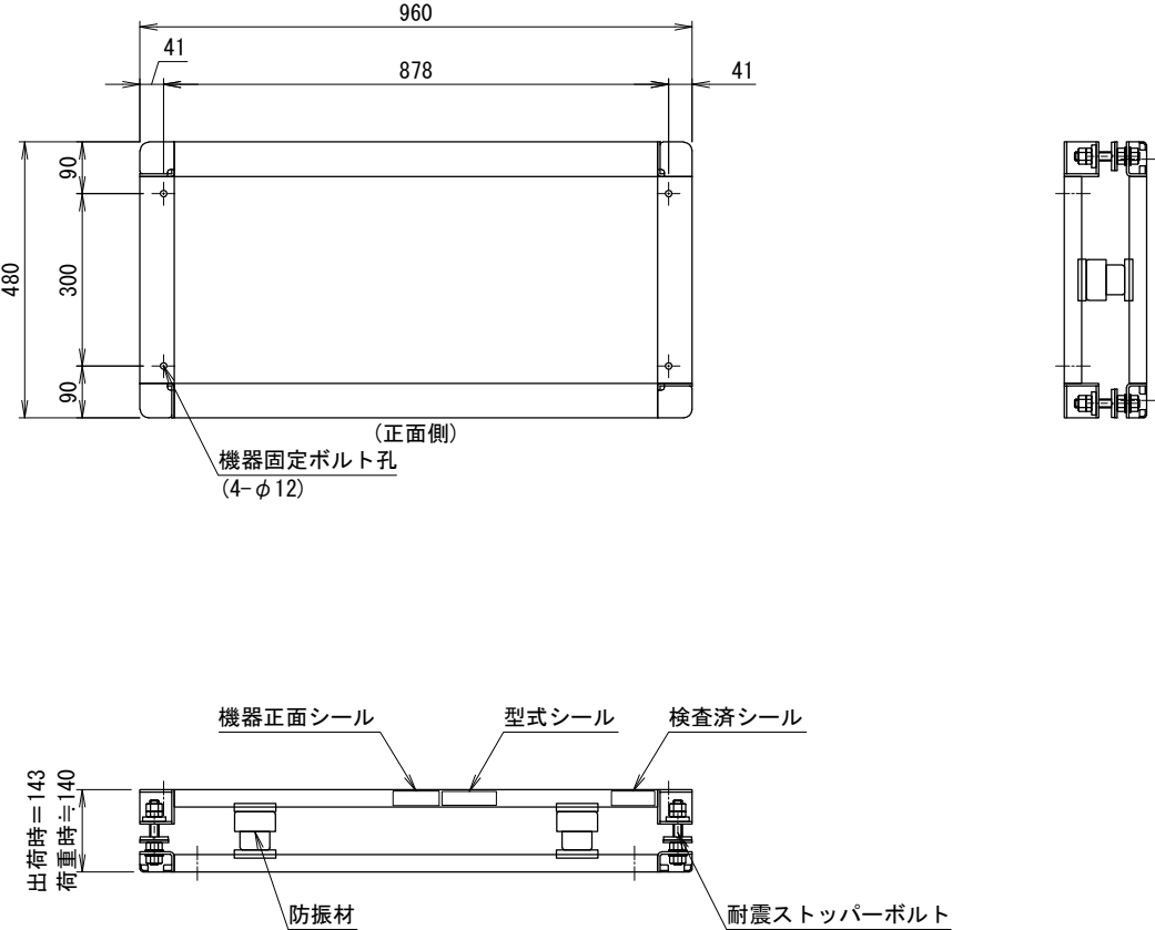
＜アンカー＞(参考) 接着系アンカー(M10) 有効埋込：80mm以上
