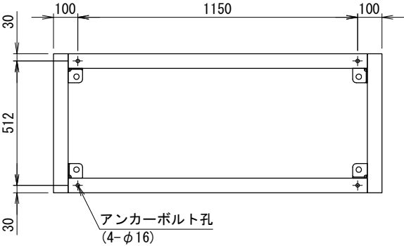
＜アンカー寸法図＞ SCALE= 1:15
