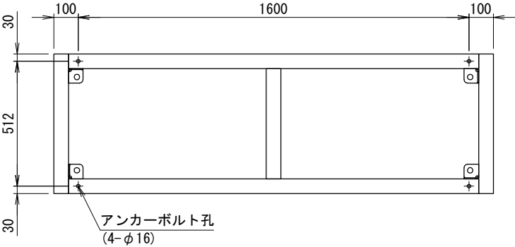
＜アンカー寸法図＞ SCALE= 1:15
